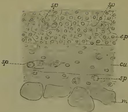
Fig. 74. Schnitt durch die Haut der Laube ( Alb. lucidus [nach Thélohan]). sp = Sporen von Myx. dispar. ep = Epithelzellen. cu = Cutis. m = Muskeln.
